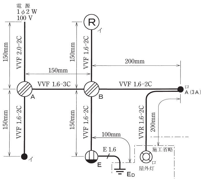
図 1 配線図
